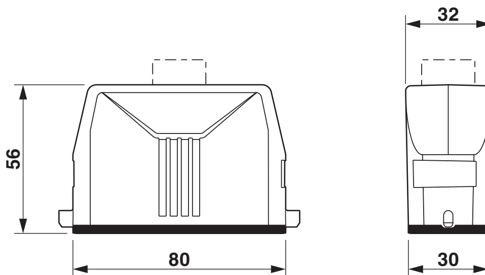
Rysunek wymiarowy
