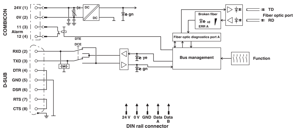
Schemat blokowy
