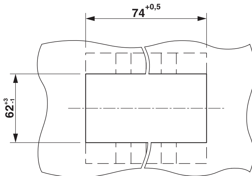
Rysunek wymiarowy
