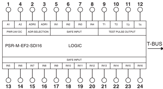
Schemat blokowy
