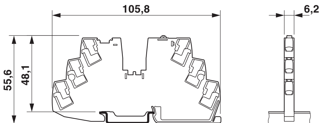
Rysunek wymiarowy
