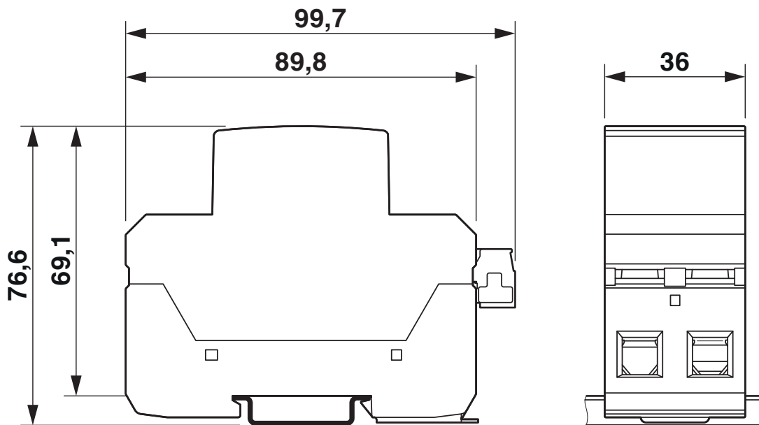
Rysunek wymiarowy
