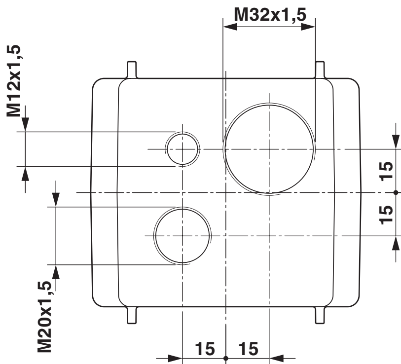
Rysunek wymiarowy
