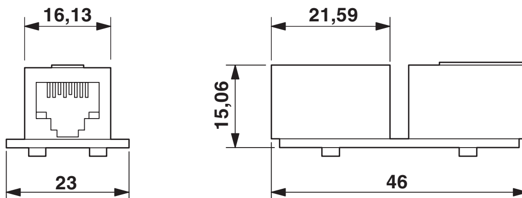
Rysunek wymiarowy
