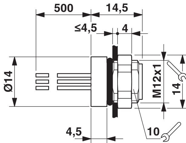
Rysunek wymiarowy
