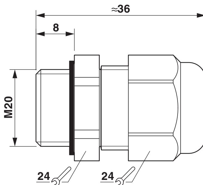
Rysunek wymiarowy
