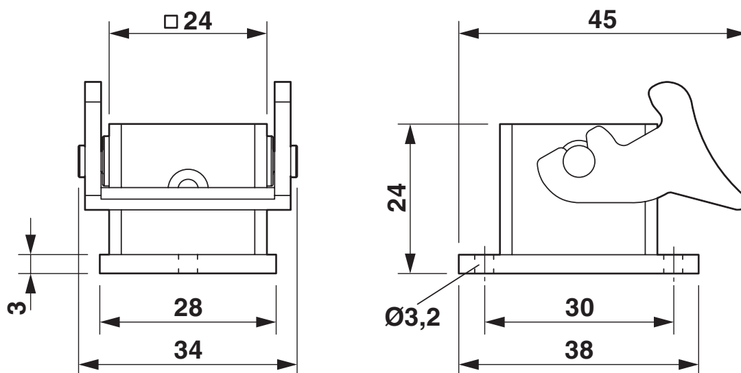
Rysunek wymiarowy
