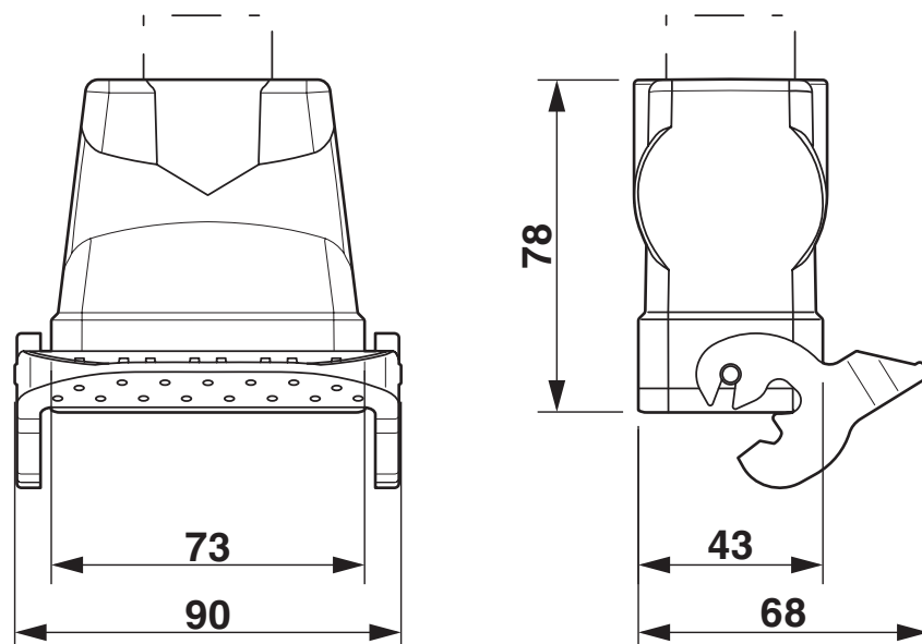
Rysunek wymiarowy
