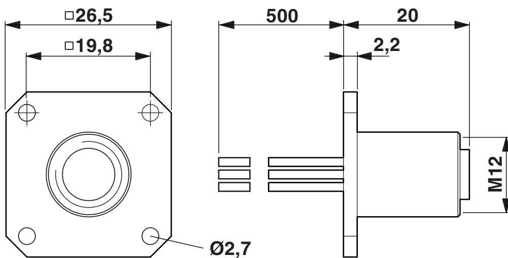
Rysunek wymiarowy
