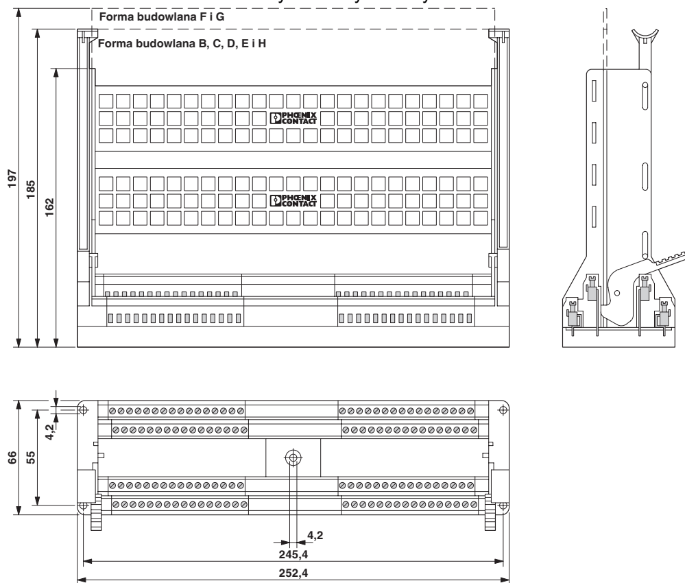
Rysunek wymiarowy
