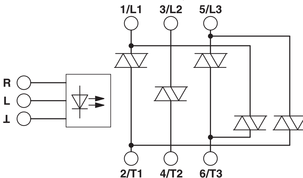
Schemat blokowy
