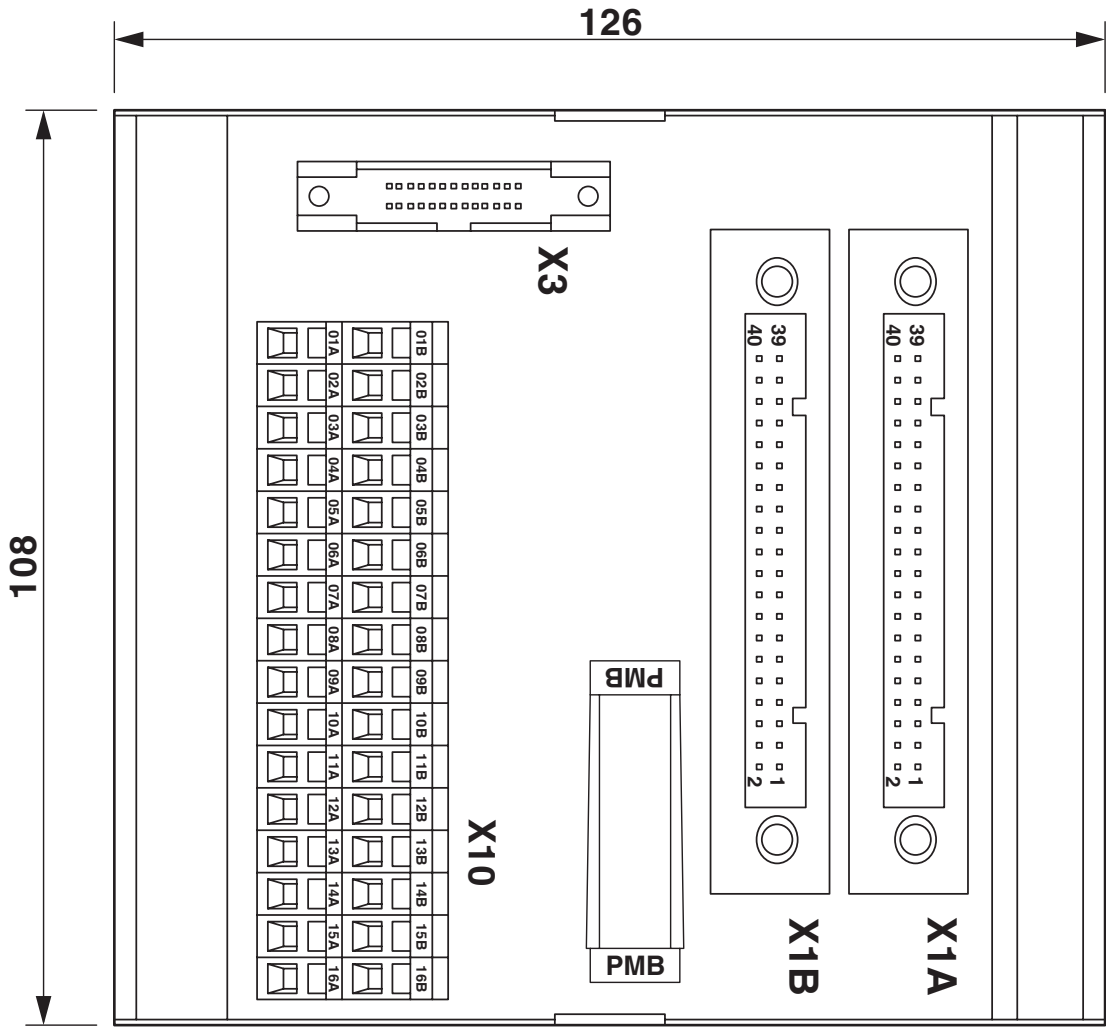
Rysunek wymiarowy
