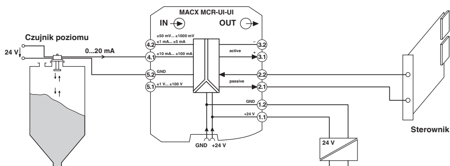
rysunek aplikacji
