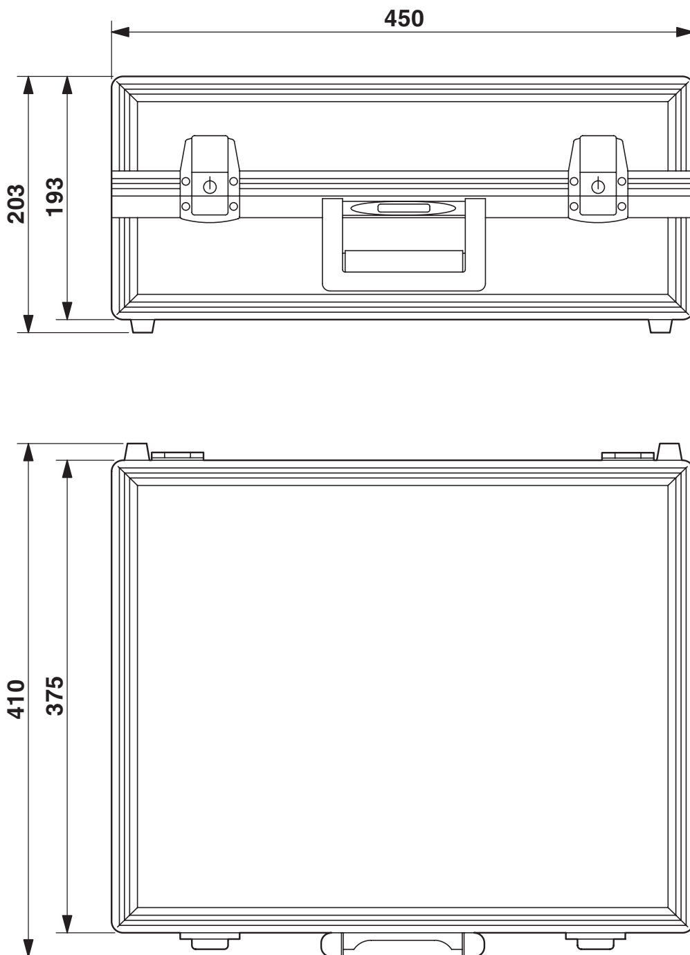
Rysunek wymiarowy
