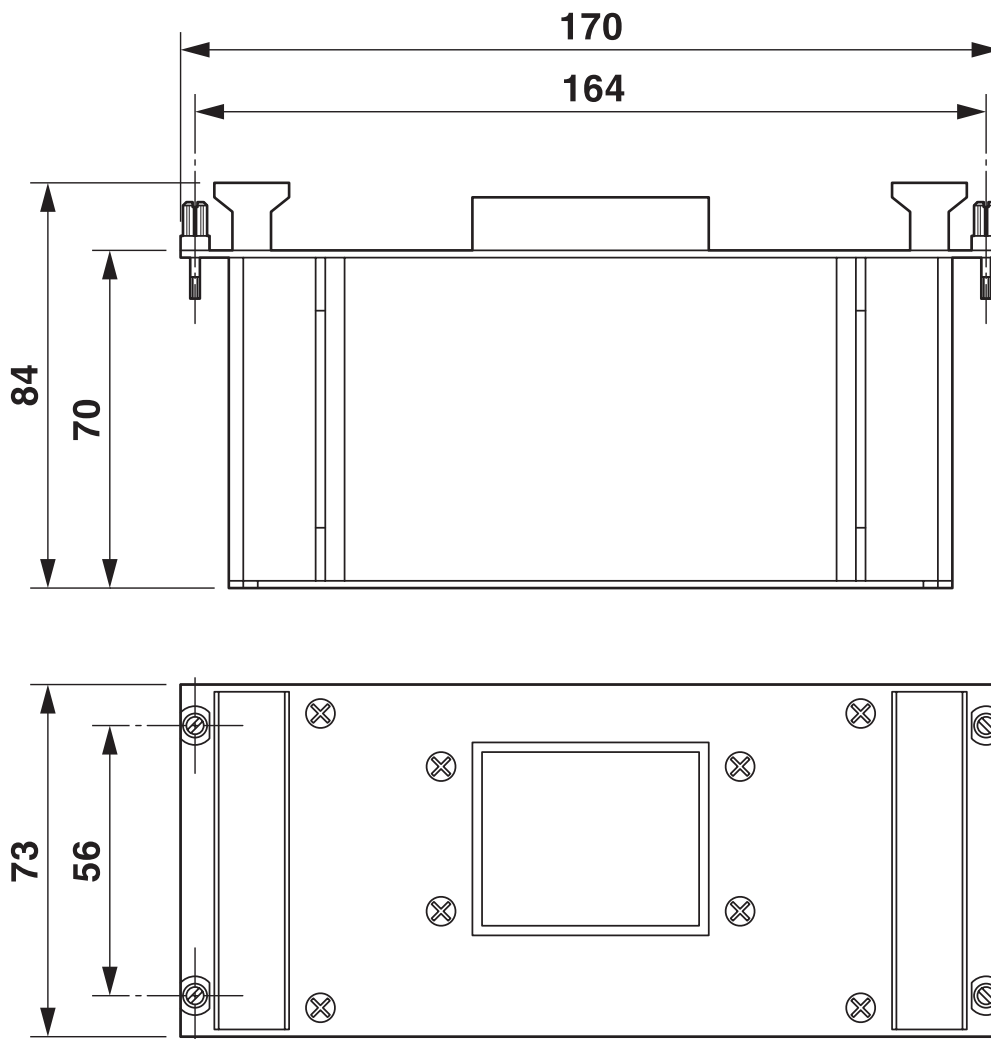
Rysunek wymiarowy
