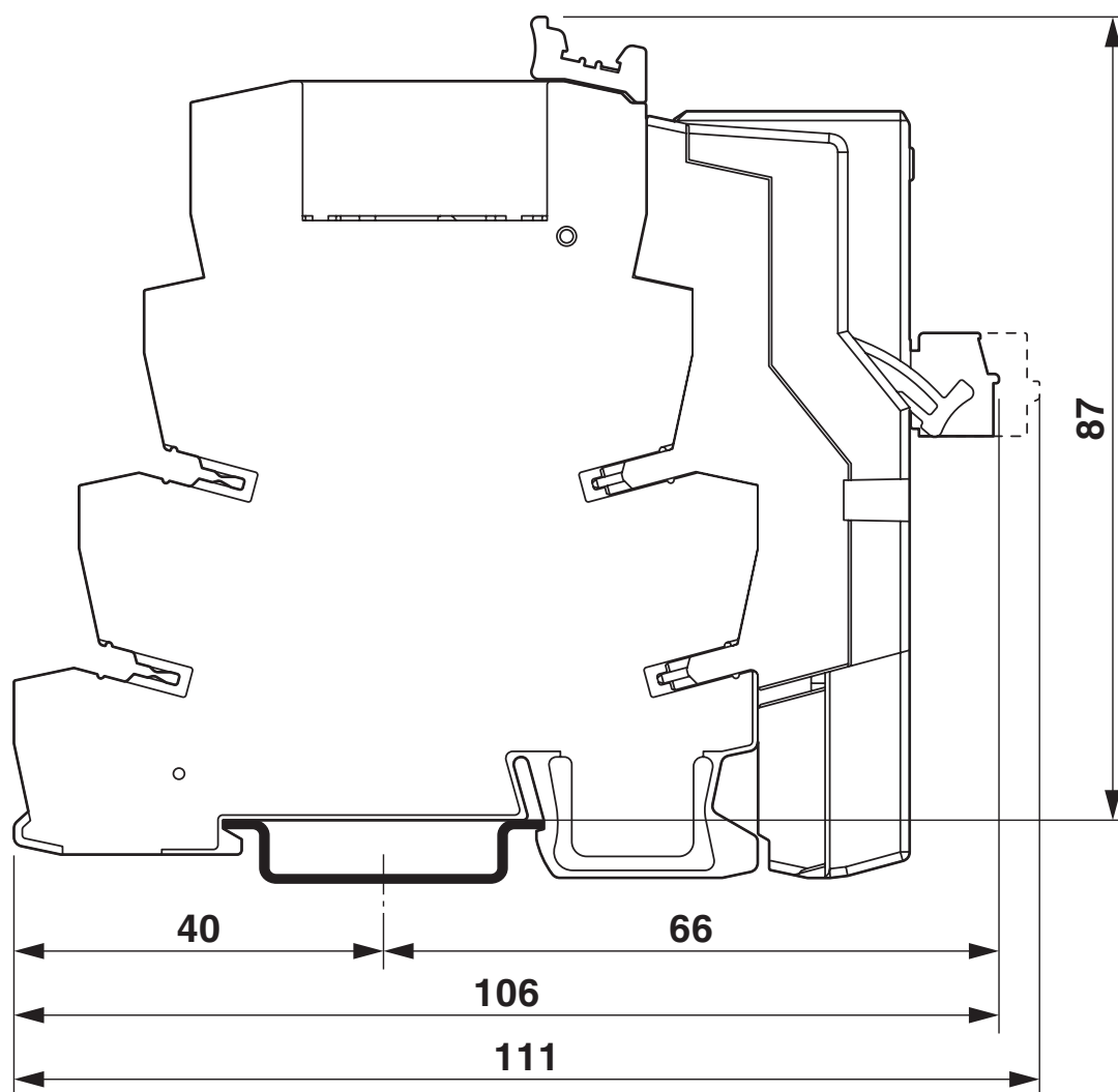
Rysunek wymiarowy
