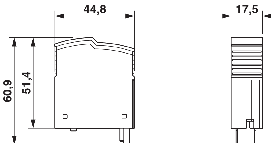
Rysunek wymiarowy
