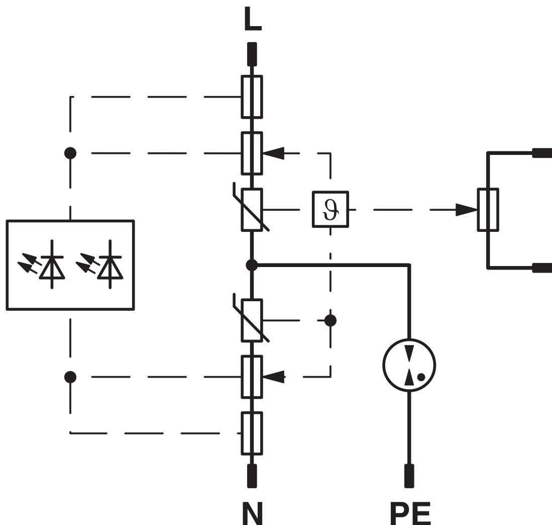
Schemat
