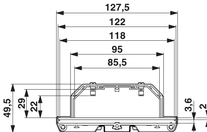
Rysunek wymiarowy
