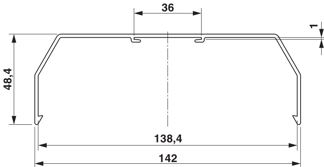
Rysunek wymiarowy
