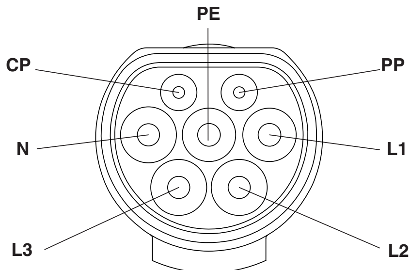
Rysunek schematyczny
