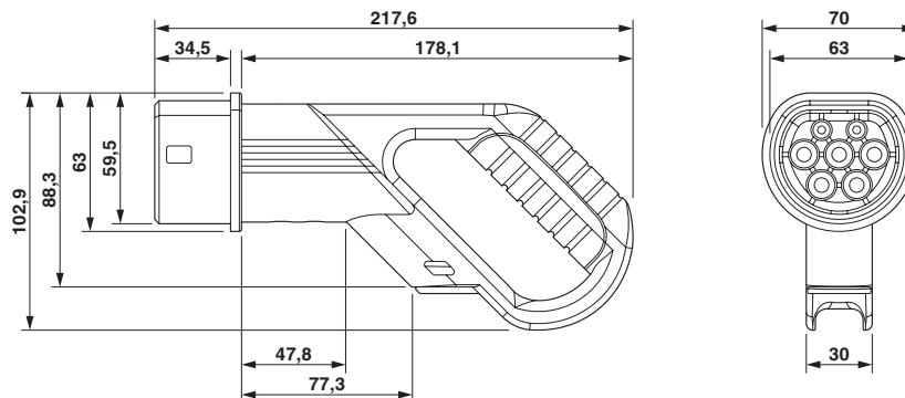
Rysunek wymiarowy
