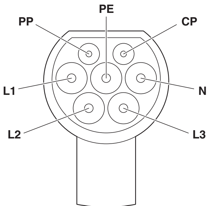
rysunek złączy
