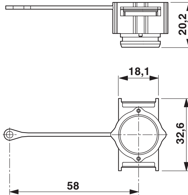
Rysunek wymiarowy
