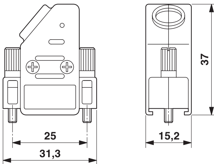
Rysunek wymiarowy
