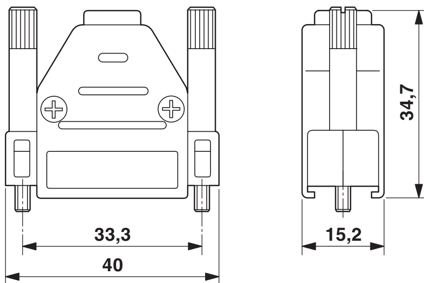
Rysunek wymiarowy
