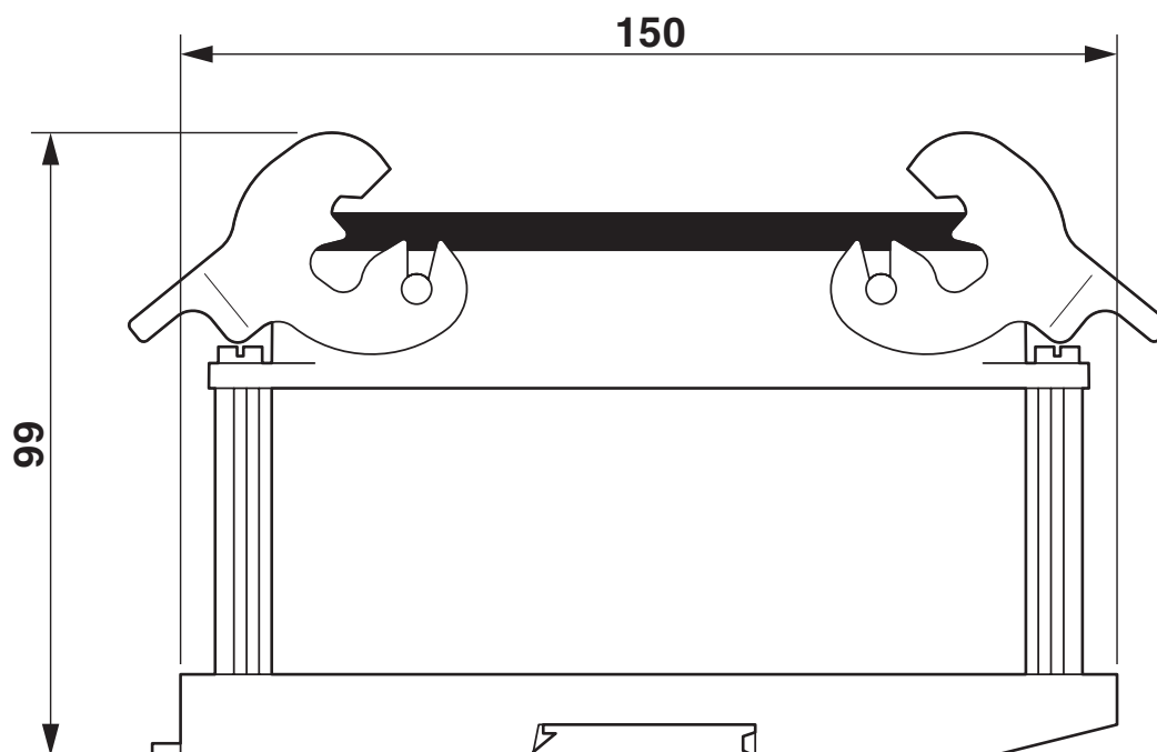
Rysunek wymiarowy
