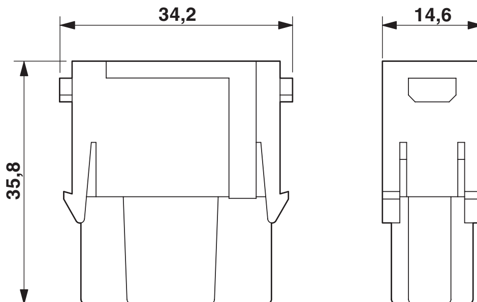
Rysunek wymiarowy
