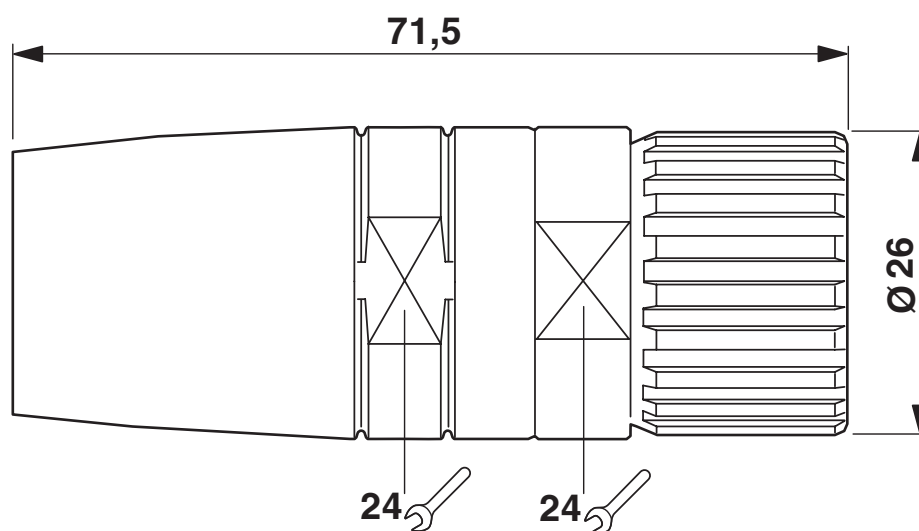
Rysunek wymiarowy
