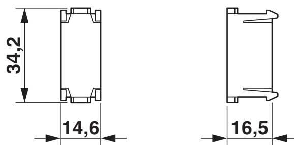
Rysunek wymiarowy
