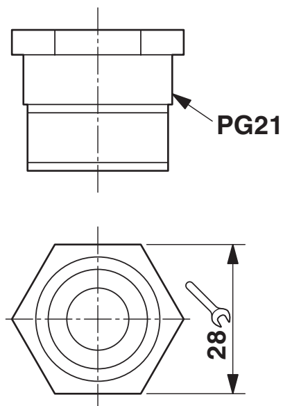
Rysunek wymiarowy
