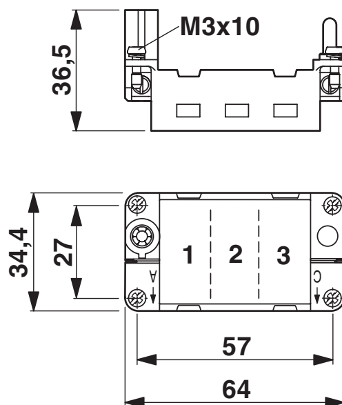
Rysunek wymiarowy
