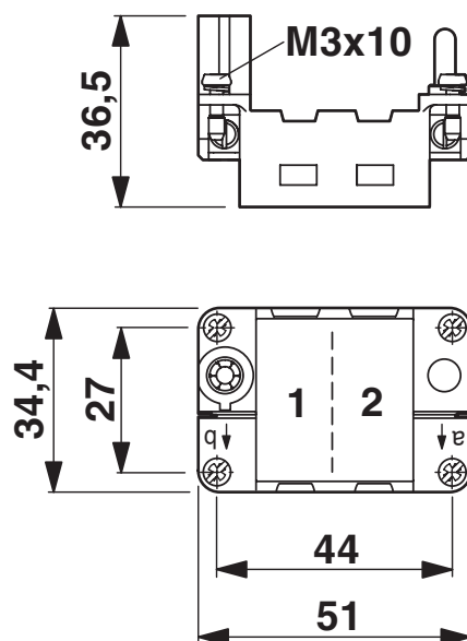
Rysunek wymiarowy
