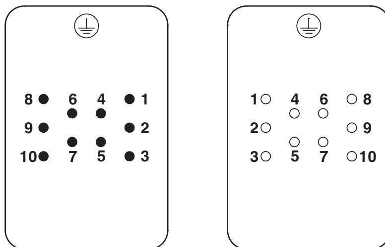
Rysunek schematyczny
