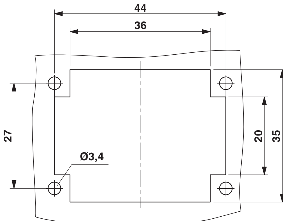
Rysunek wymiarowy
