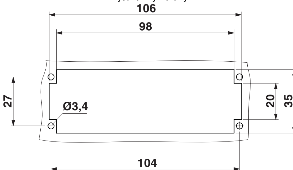
Rysunek wymiarowy
