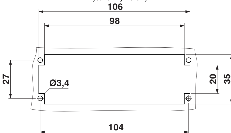
Rysunek wymiarowy
