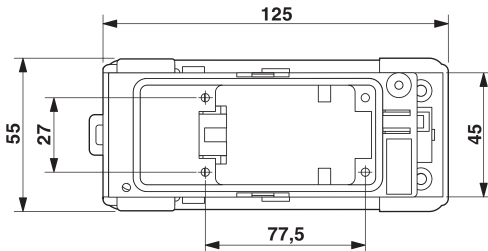
Rysunek wymiarowy
