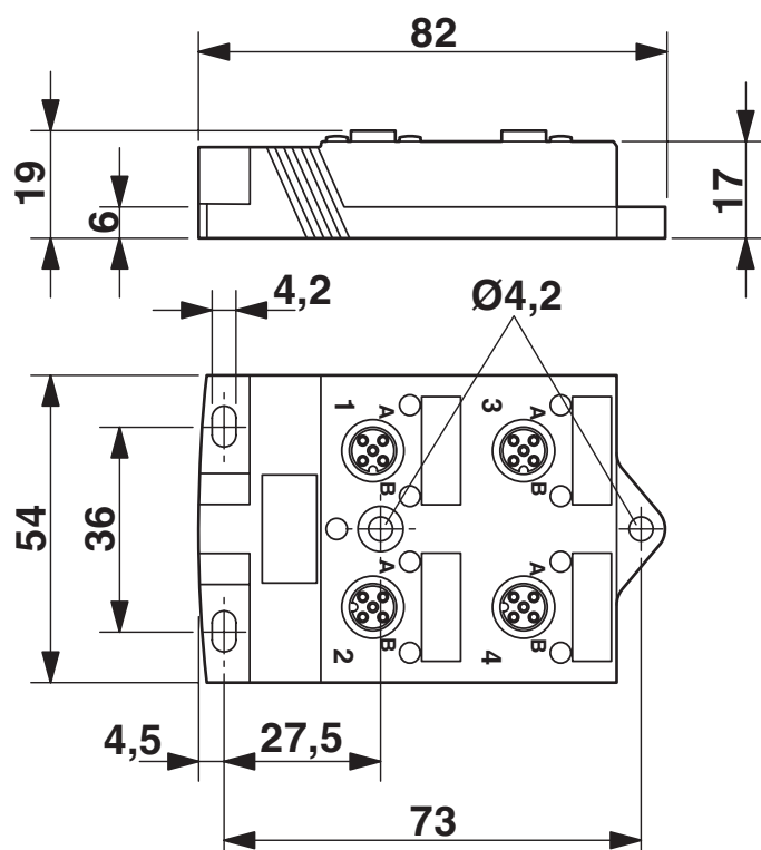
Rysunek wymiarowy
