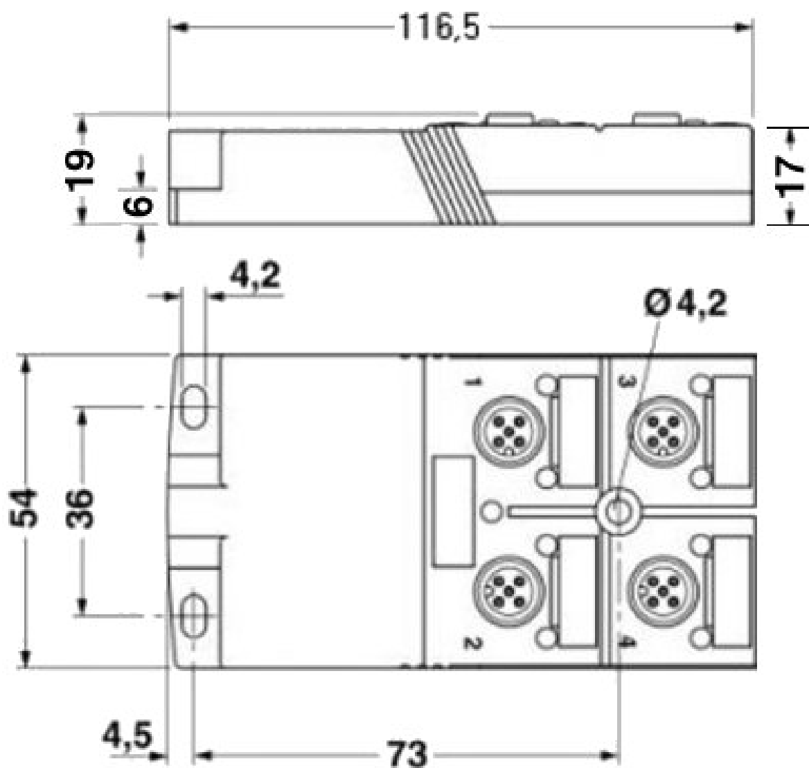
Rysunek wymiarowy
