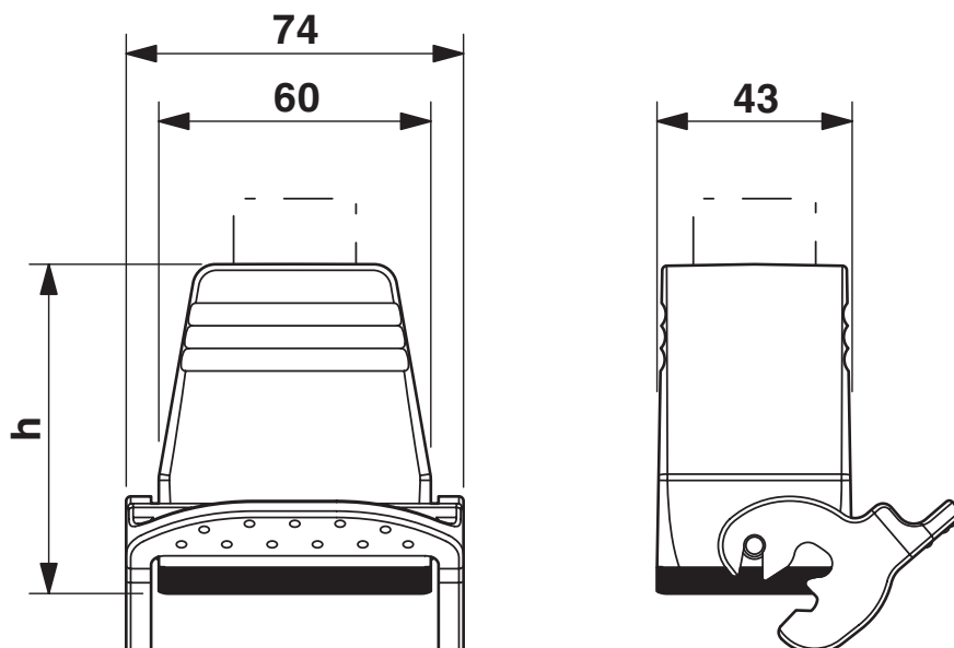
Rysunek wymiarowy
