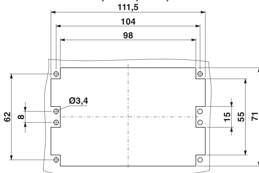
Rysunek wymiarowy
