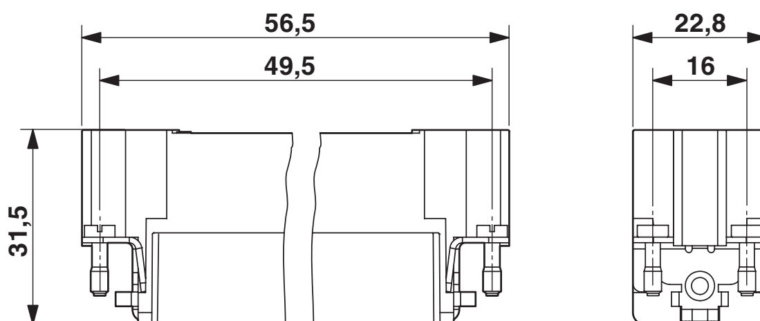
wkładka styku męskiego (styki toczone)
