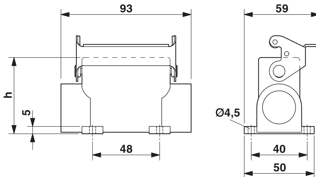
Rysunek wymiarowy
