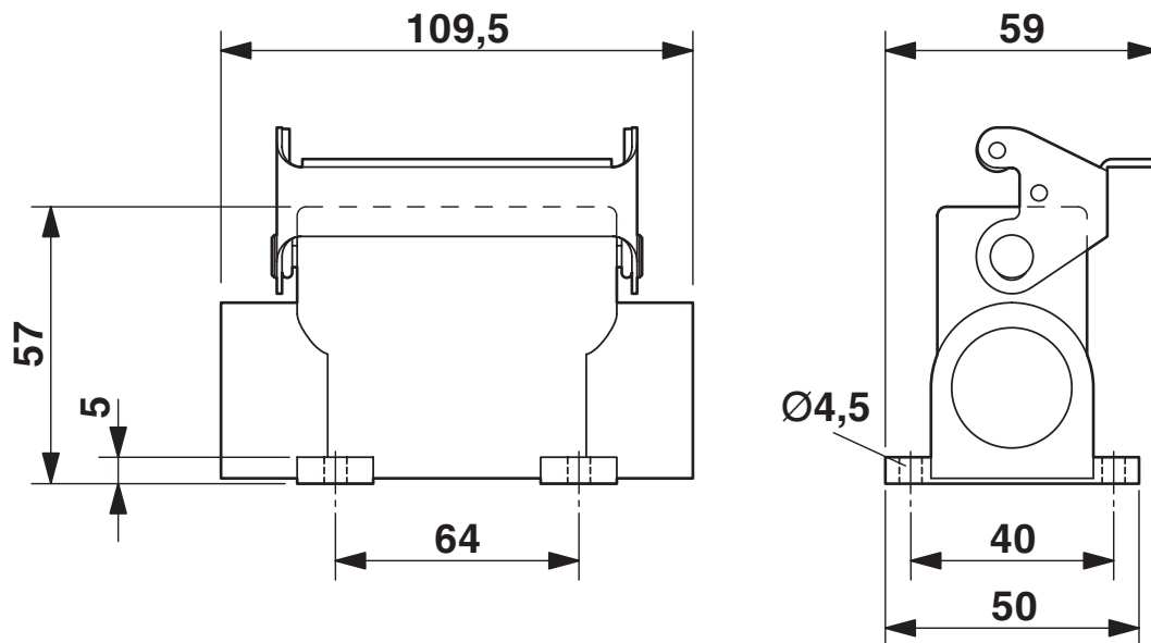
Rysunek wymiarowy
