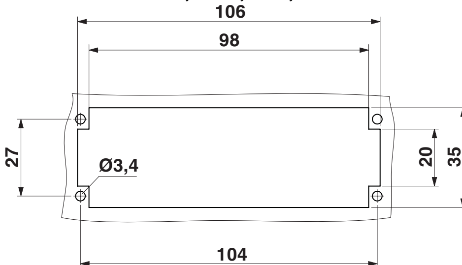
Rysunek wymiarowy
