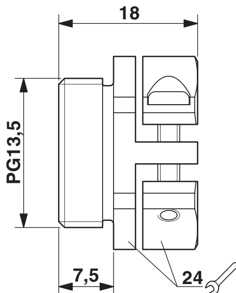
Rysunek wymiarowy
