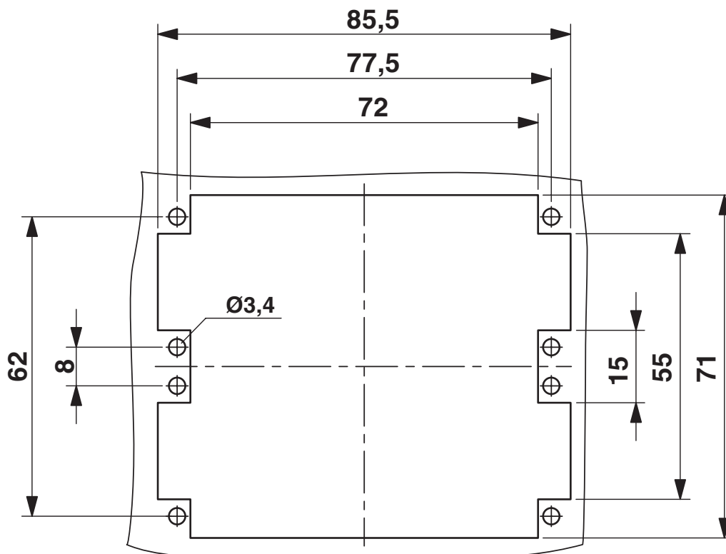
Rysunek wymiarowy
