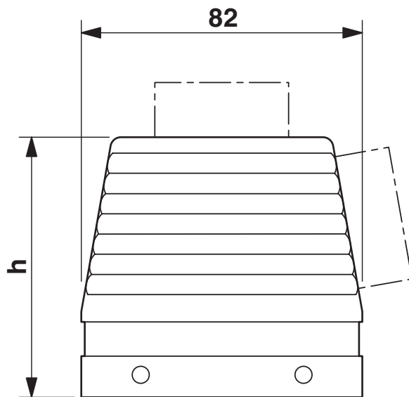
Rysunek wymiarowy
